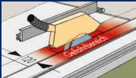
Spaltkeil, Schutzhaube und Tischverlängerung
