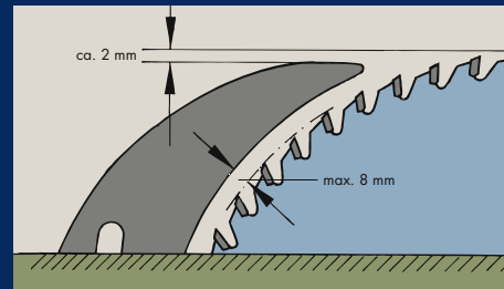
Spaltkeileinstellung für verdeckte Sägeschnitte
